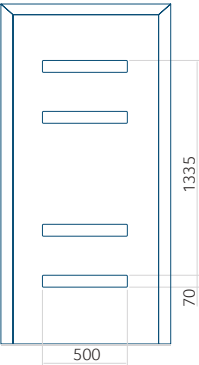
Technische Zeichnung
