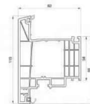
HO8540 AUßEN ÖFNEND
