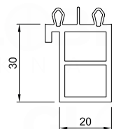
416 139 für Bautiefe 76 mm
