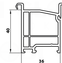
NP0400 für Bautiefe 82 mm
