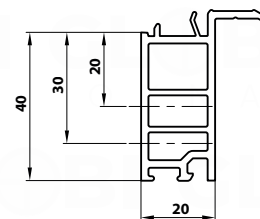
NP0370 für Bautiefe 82 mm
