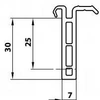
NP0320 für Bautiefe 82 mm
