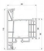
AUßEN ÖFNEND HO8540
