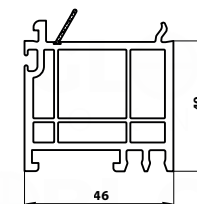
416 146 für Bautiefe 76 mm
