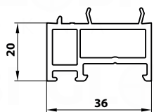
NP0200 für Bautiefe 82 mm
