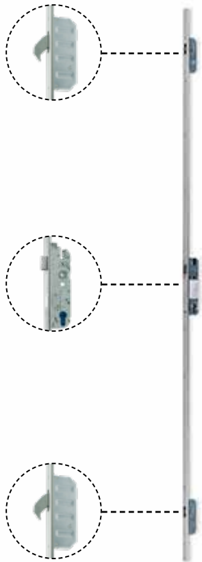
Winkhaus 3-fach-Hakenverriegelung (Standard in der SL75-Serie)
