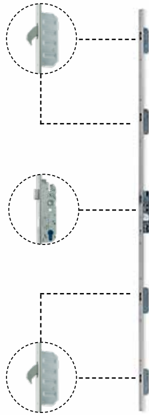
Winkhaus 5-fach-Hakenverriegelung (Standard in der P90-Serie)
