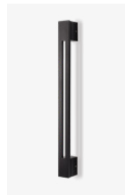
VP-35 Ø40 mm x 10 mm, einseitig, Stahl, Farbe schwarz, gerade Stützen / une face, acier, co- uleur noire, pattes droites
