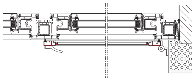
montaż na ścianie
