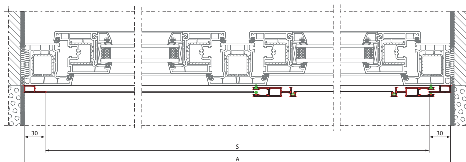
Moskitiera ramkowa przesuwna z ramą montaż we wnęce
