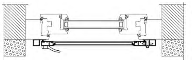
montaż na ramie okna we wnęce
