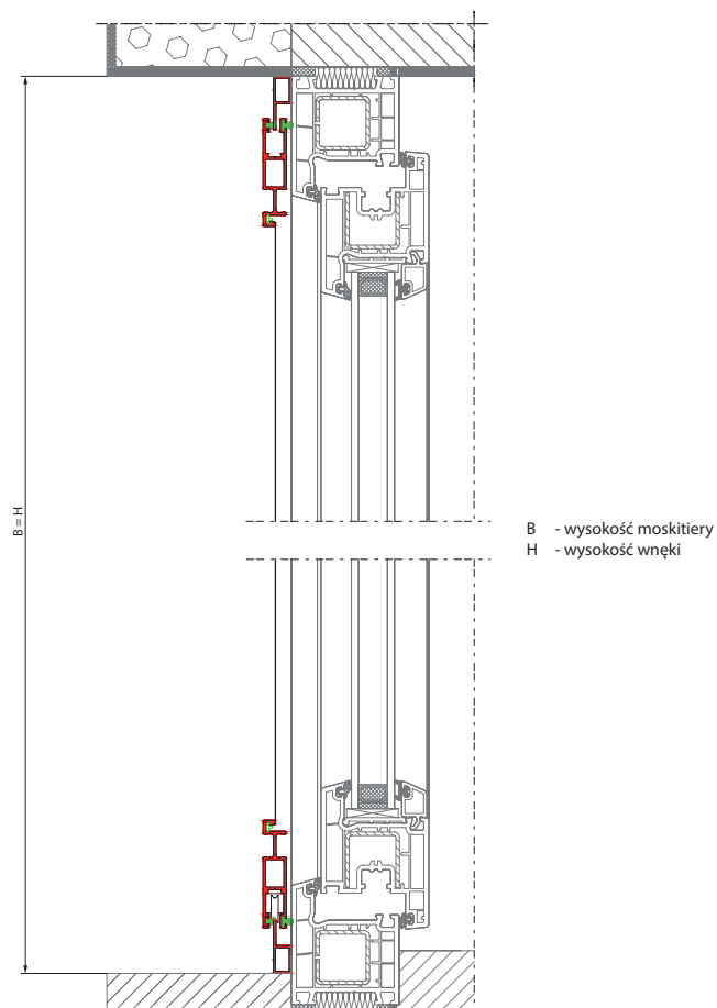
Moskitiera ramkowa przesuwna z ramą montaż we wnęce
